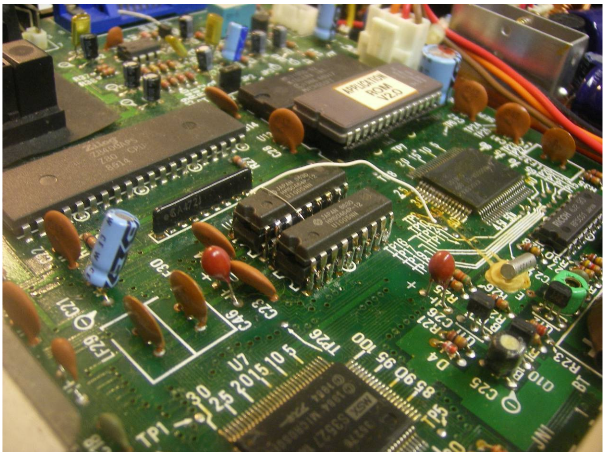
Het geheugen is geplaatst met de verbinding naar TP9
